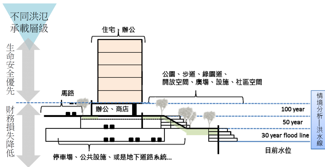
堤線調整概念示意圖
